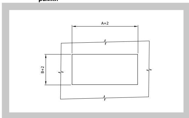
Рис. 5 Рекомендуемые размеры монтажных отверстий для жалюзи без крепительной рамки
