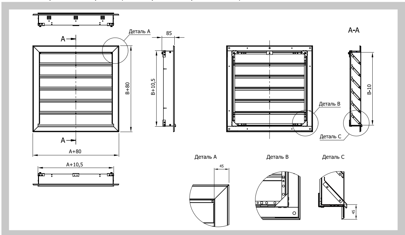
Рис. 3 С крепительной рамкой (без отверстия для присоединения)
