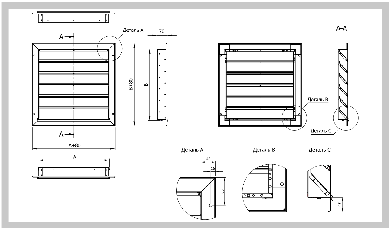
Рис. 2 Без крепительной рамки, с отверстиями для присоединения
