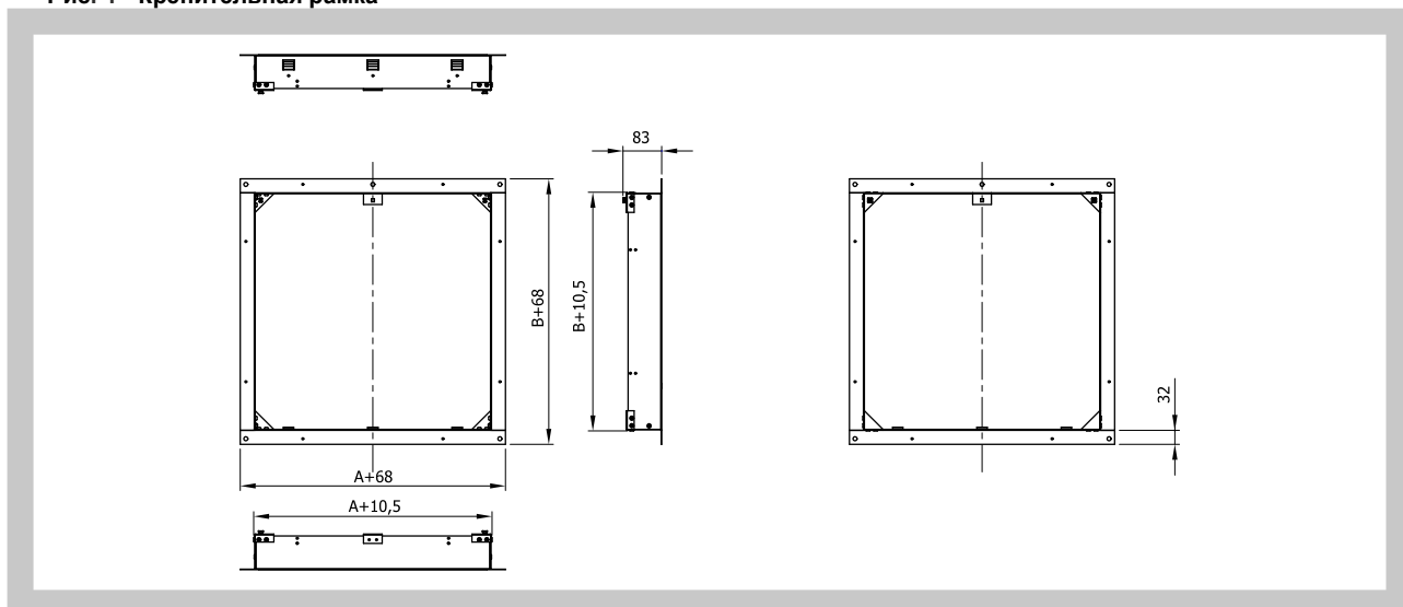
Рис. 4 Крепительная рамка
