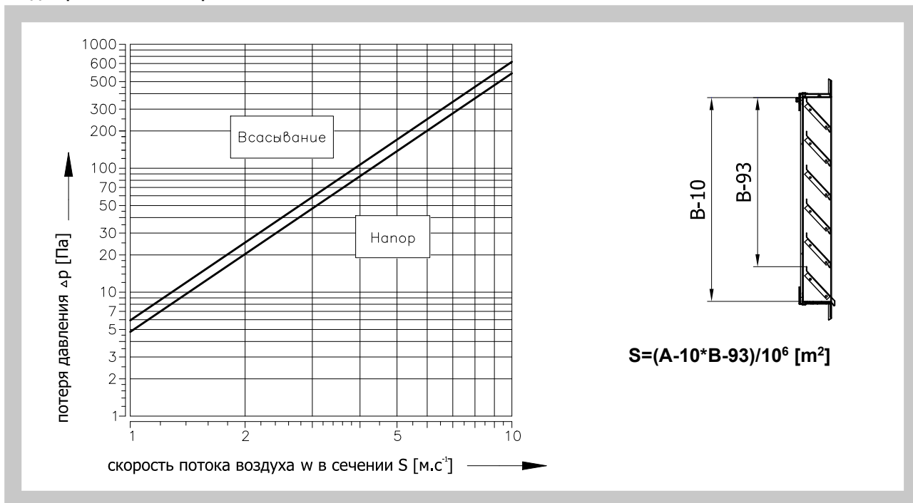
Диаграмма 5.1.1. Потеря статического давления PDZM
