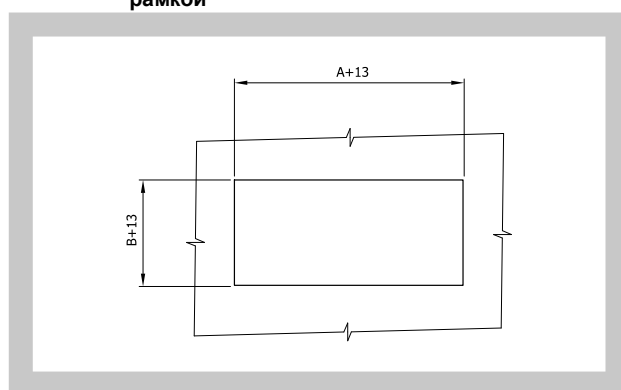
Рис. 6 Рекомендуемые размеры монтажных отверстий для жалюзи с крепительной рамкой
